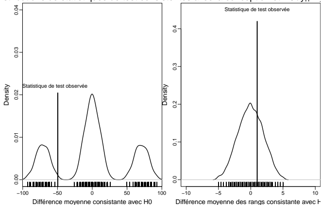
Figure 1: Utiliser la conception d'expérience pour tester une hypothèse avec deux statistiques de test différentes.
